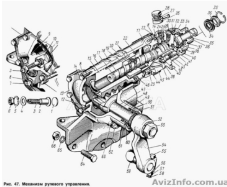
Рис. 47. Механизм рулевого управления.
